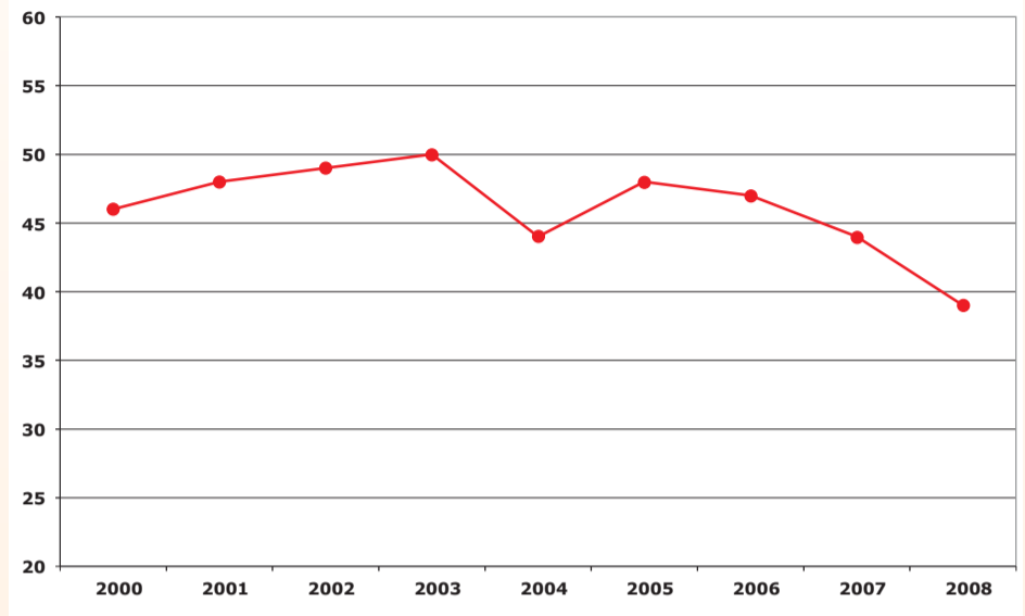
EVOLUCIÓN DE LA MEDIA ANUAL DE DIÓXIDO DE NITRÓGENO EN SANT ANDREU (2000-2008)
