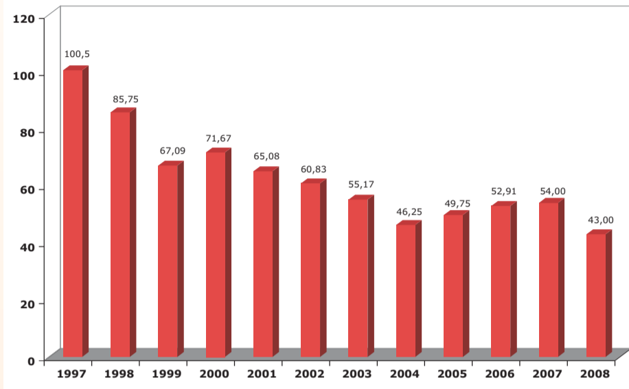
EVOLUCIÓN DE LA MEDIA ANUAL DE LAS PARTÍCULAS PM10 EN SANT ANDREU (1997-2008)
